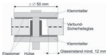
Bild 3: Prinzipskizze Querschnitt Tellerhalter
