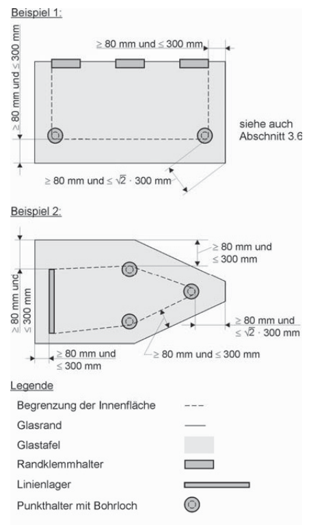
Bild 1: Prinzipskizze Glasauskragung
