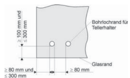
Bild 2: Randabstände Bohrloch
