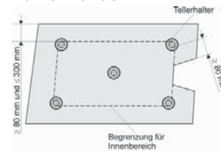
Bild 6: Innenbereich punktförmig gelagerter Überkopfverglasung
