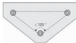
Bild 5: Prinzipskizze Winkeldefinition punktgelagerte VSG-Scheibe
